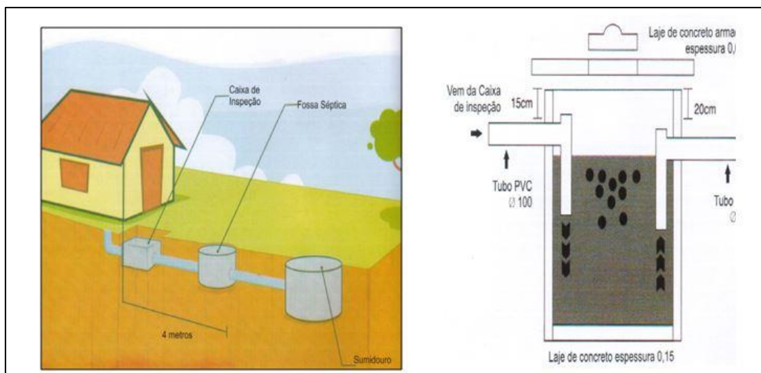
Figura 28 - Sistema Individual de Tratamento – Fossas Sépticas.
