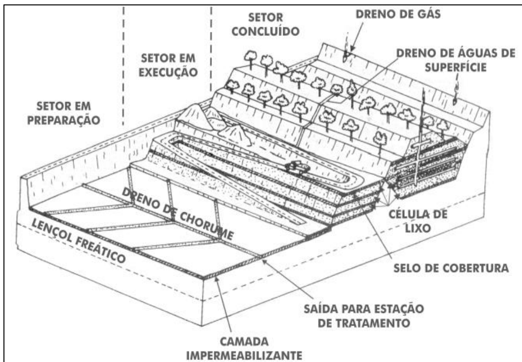
Figura 99 - Projeto técnico de aterro sanitário.
