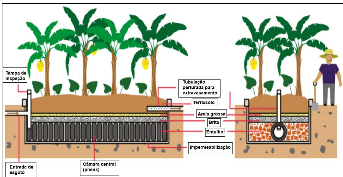
Figura 82 - Esquema de BET.
