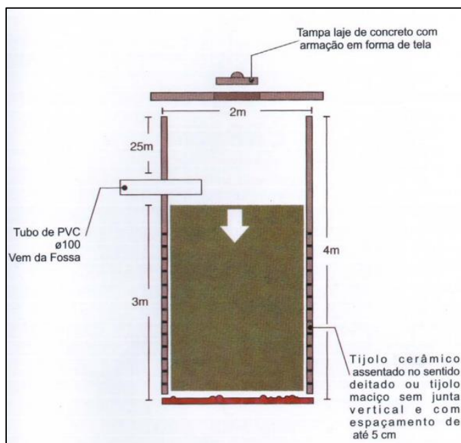
Figura 74 – Sistema individual de tratamento – Sumidouro.
