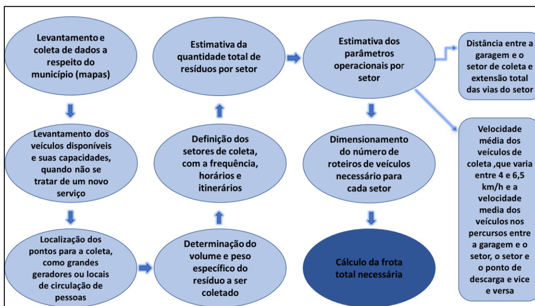
Figura 85 - Fluxograma das etapas mínimas do dimensionamento da coleta convencional.
