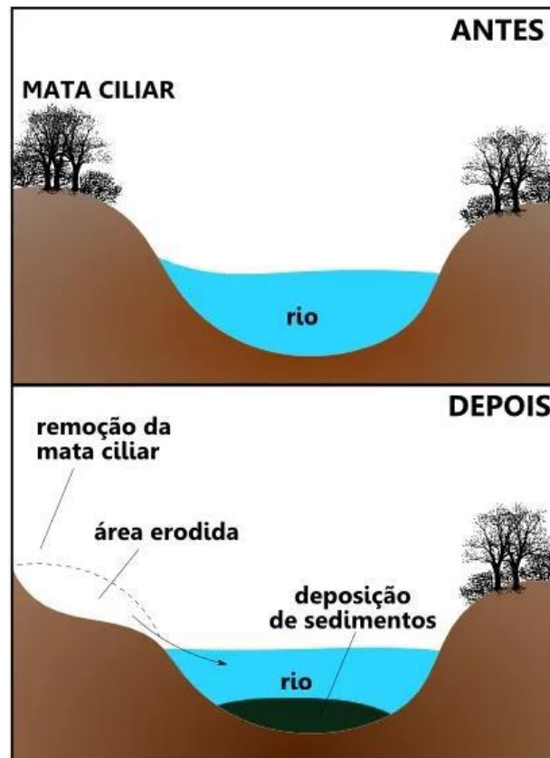
Figura 110 - Esquema de Assoreamento.
