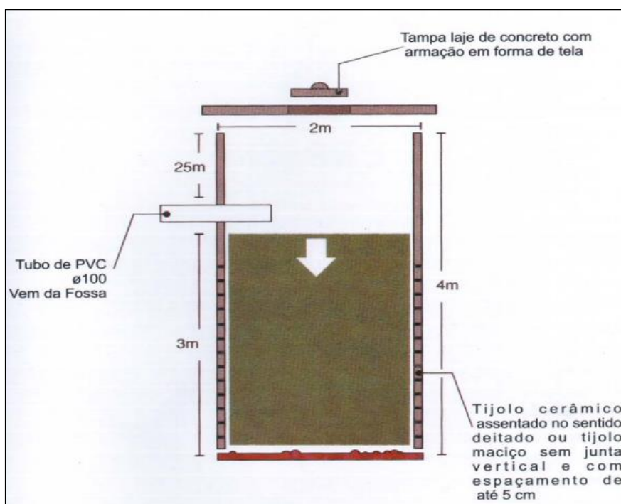
Figura 30 – Sistema individual de tratamento – Sumidouro.
