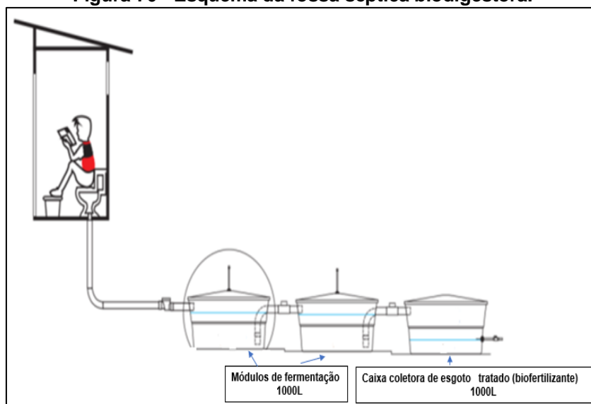
Figura 76 - Esquema da fossa séptica biodigestora.
