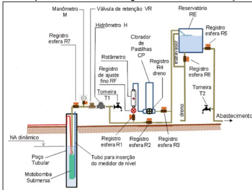
Figura 19 - Esquema de tratamento de água subterrânea com cloração simples.
