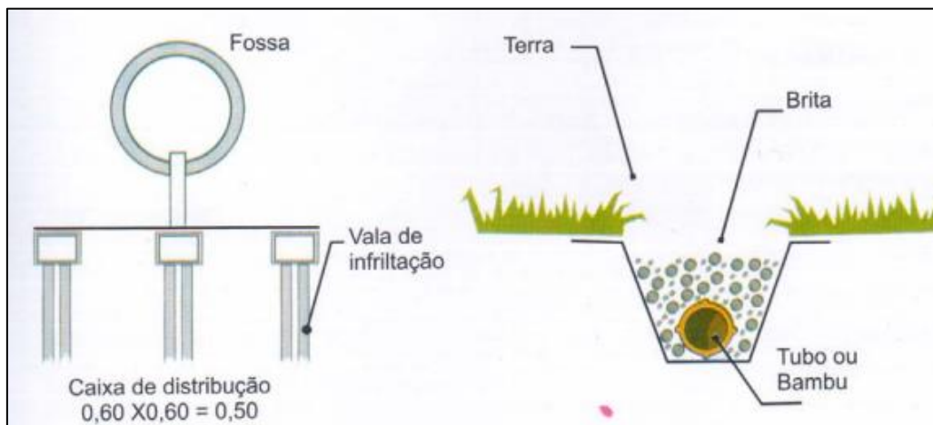
Figura 73 – Sistema de tratamento individual – Valas de Infiltração.
