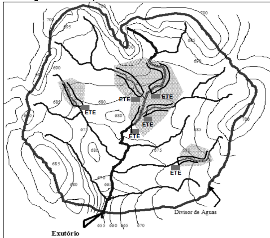
Figura 69 - Exemplo de sistema descentralizado.
