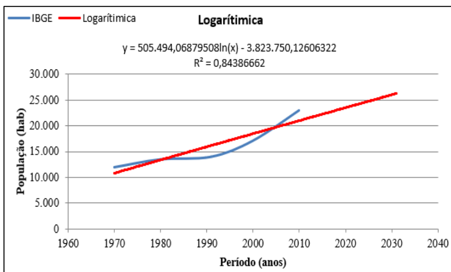
Gráfico 11 - Análise comparativa entre o crescimento populacional pelo IBGE e a Curva Logarítmica.
